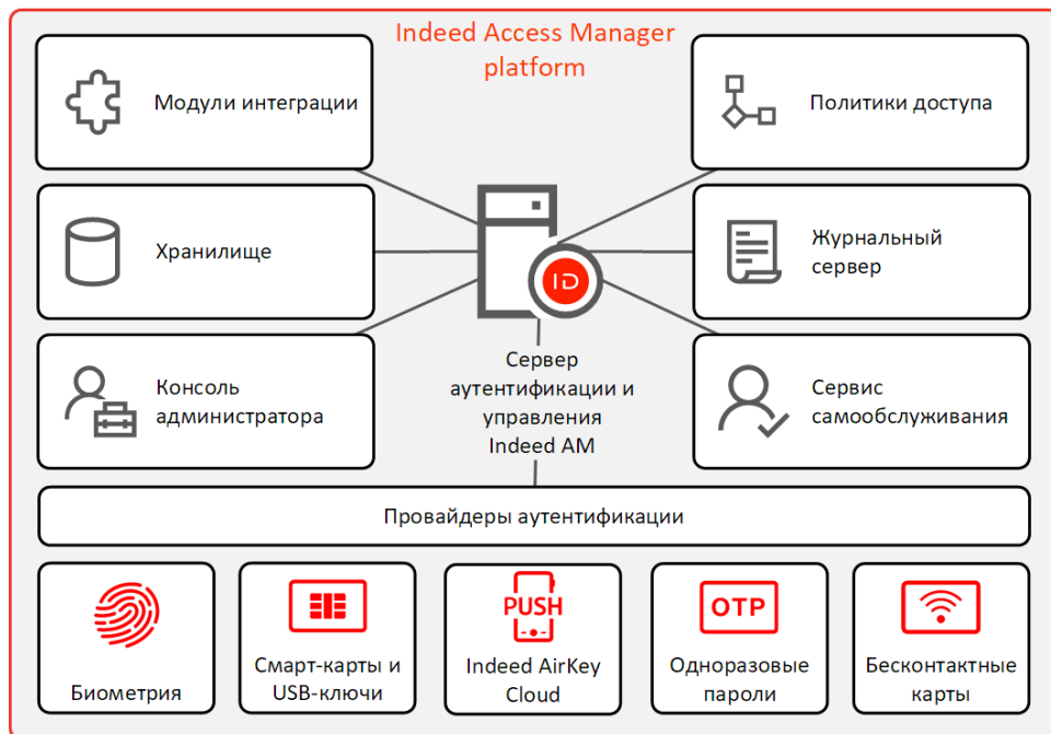
Рисунок 1. Платформа Indeed Access Manager
